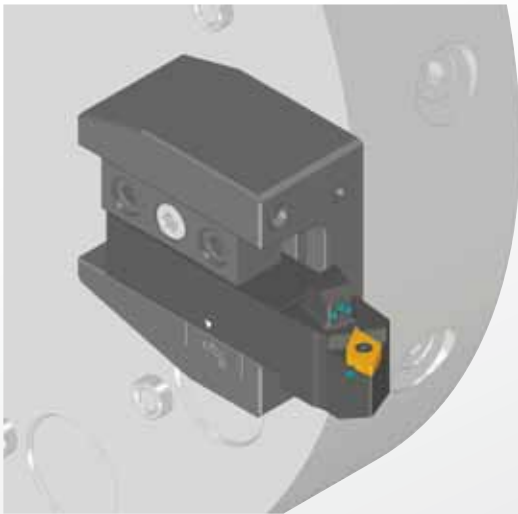
Längsdrehhalter für Scheibenrevolver
