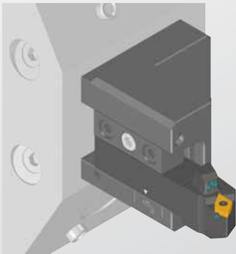
Längsdrehhalter für Sternrevolver
